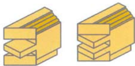
Mitre Joint
